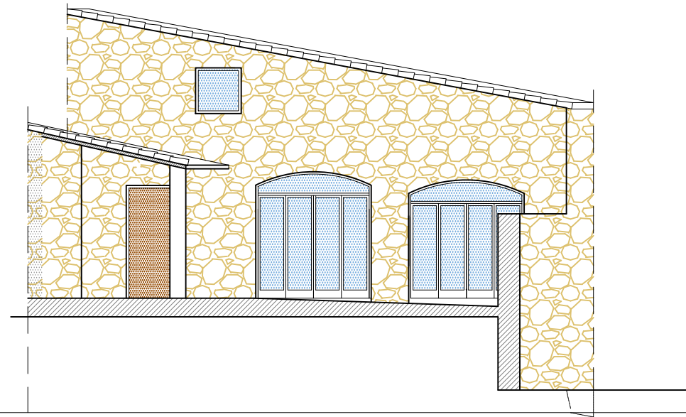
ALÇAT D — FAÇANA PATI CONSTRUCCIÓ AUXILIAR
