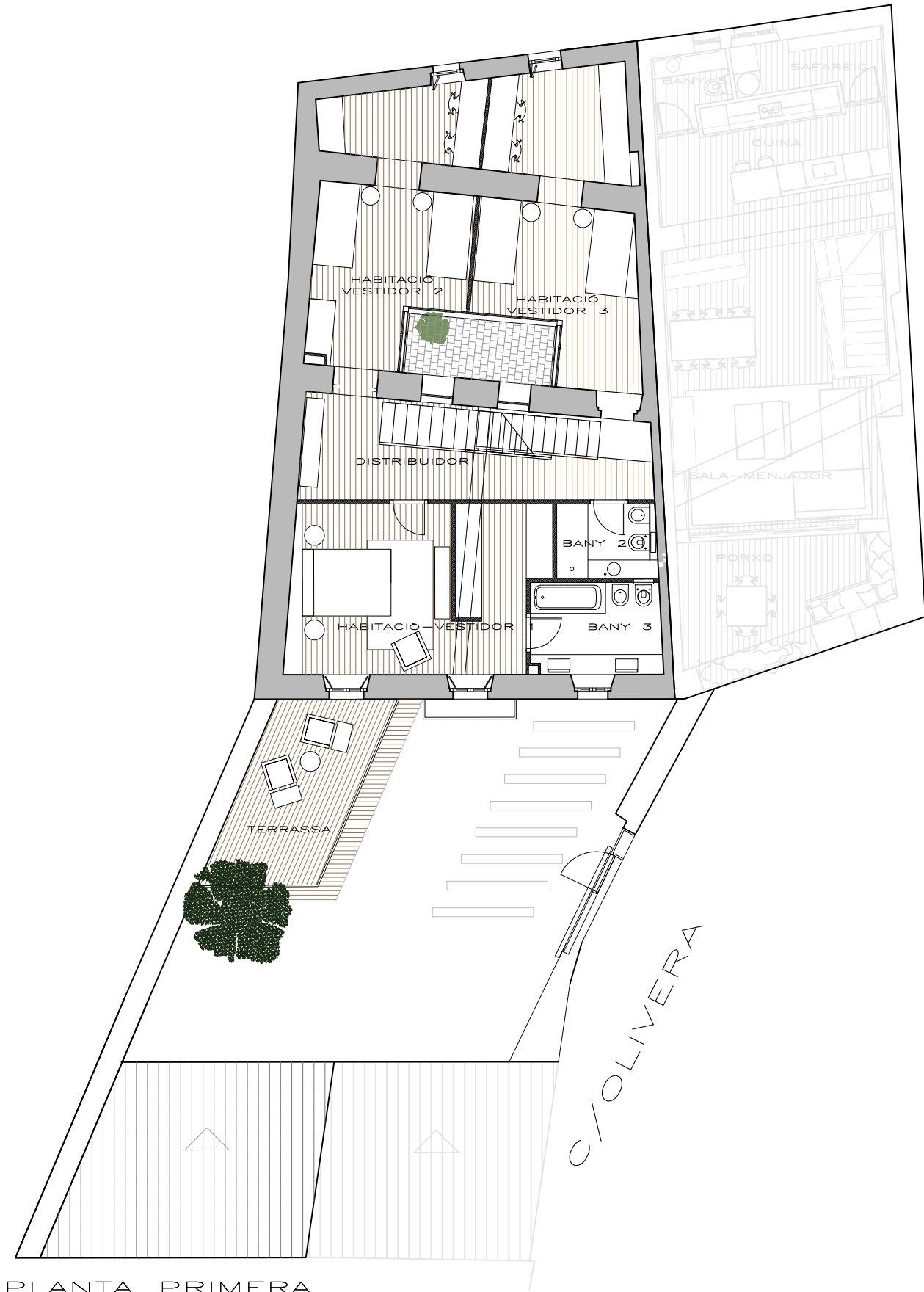
PLANTA PRIMERA
